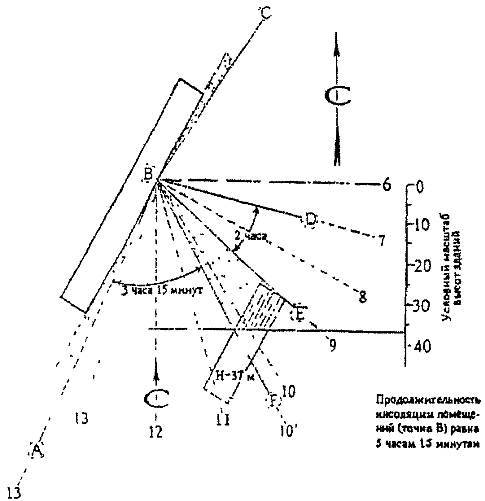
Рис. 5. Схема определения инсоляции.
