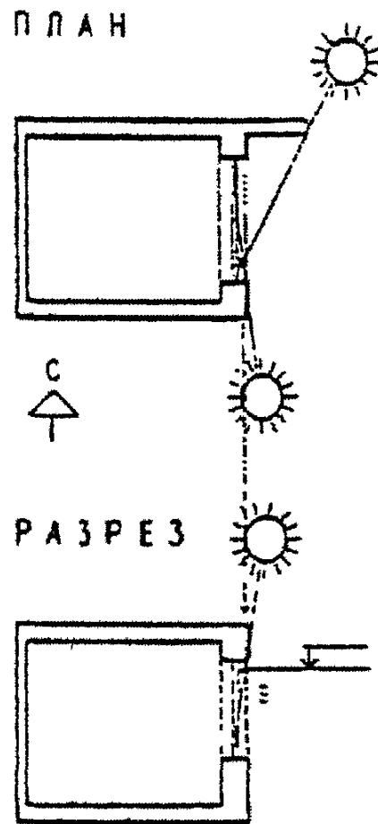
Рис. 4. Схема определения расчетной точки для окна с примыкающей стеной.
