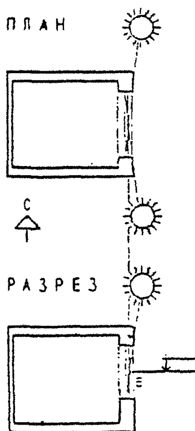
Рис. 1. Схема определения расчетной точки для окна.
